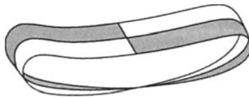
Möbius band
